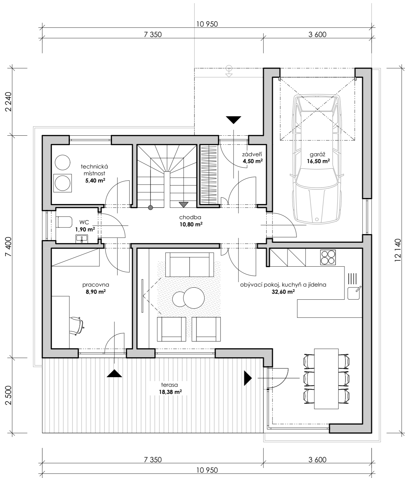
půdorys 1.NP
