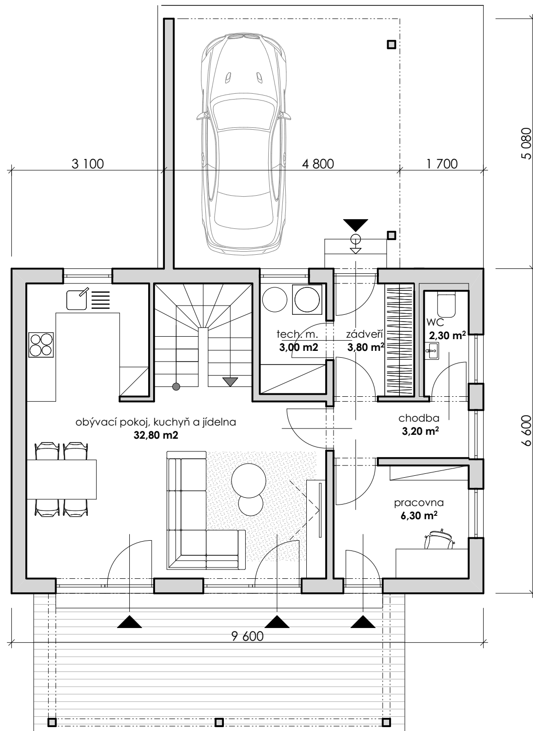
půdorys 1.NP
